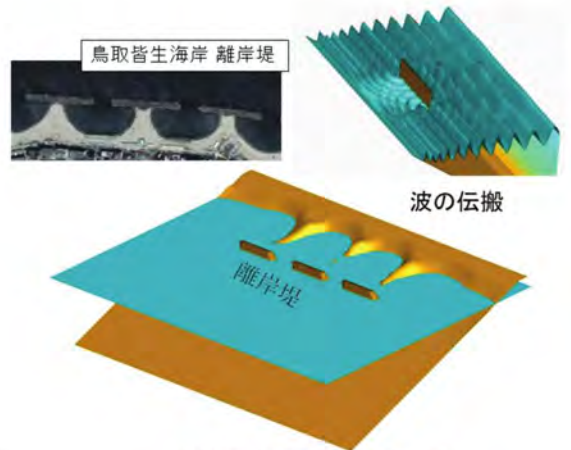
3次元海浜変形予測モデル シミュレーション例(トンボロの発達)
