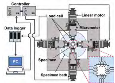
二軸引張試験装置を活用した生体材料の力学実験
