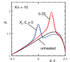
局所加熱マイクロ滑流路内の空気膜圧力分布
