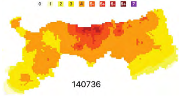
2016年10月鳥取県中部の地震における、緊急地震速報警報（第3報）配信時の震度分布（データを元に再現）
