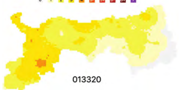
2018年4月鳥根県西部の地震において把握された最終震度分布
