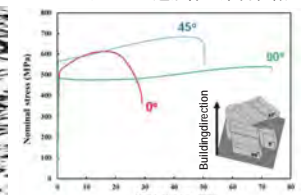
ステンレス鋼の応力-ひずみ曲線
