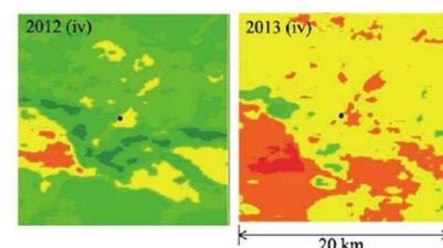
2012年(左)と2013年(右)夏のNDVI(正規化植生指数)。2012年は多雨の影響で産地の植生量が多かった(Gantsetseget et al. 2017)。
