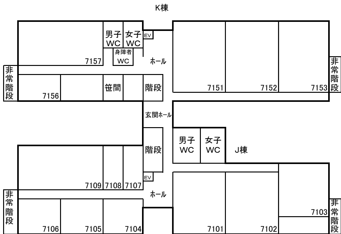
1 階 平 面 図
