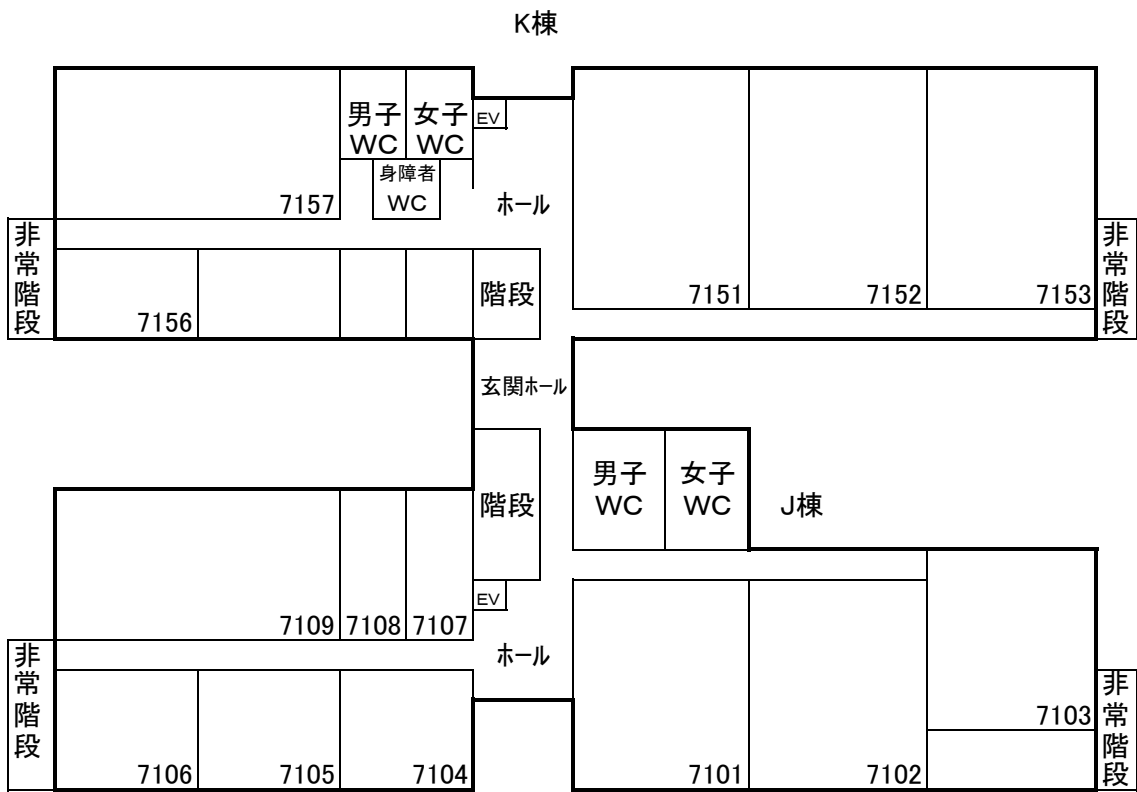
1 階 平 面 図
